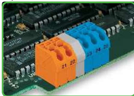
Маркировка самоклеющимися маркировочными полосками или путем непосредственной печати. Клеммные колодки различных цветов (с/без разделителя) доступны по запросу.
