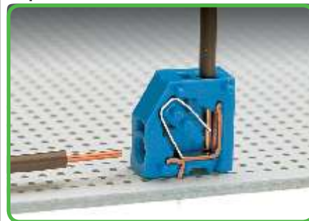
Вставка одножильного проводника путем вставки. Горизонтально или вертикально.
