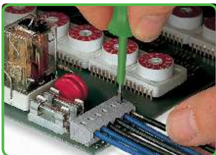
Извлечение проводника при помощи отвертки. Клеммная колодка без нажимных кнопок.
