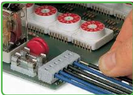
Вставка одножильного проводника путем вставки. Клеммная колодка без нажимных кнопок.
