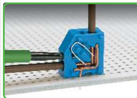
Извлечение проводника при помощи 2,5 мм отвертки.
