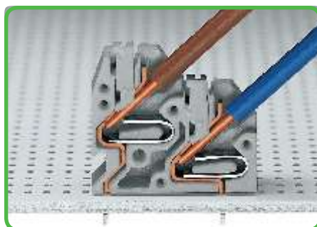
Компактный монтаж. Подключение одножильных проводников путем вставки.
