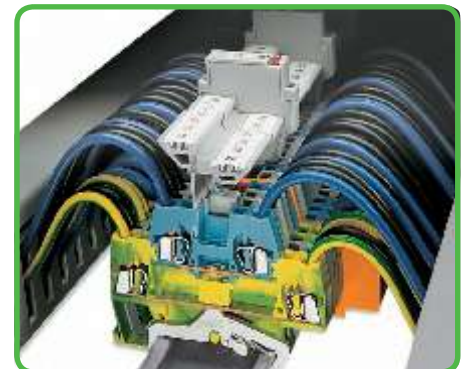
Пример двухуровневой клеммной сборки смешанного монтажа.
