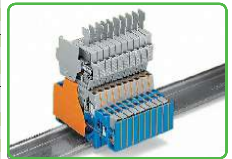
Монтаж двухуровневой клеммы с предохранителями.
