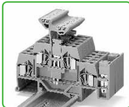
Объединение вертикальными и поперечными перемычками.
