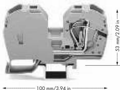
Заделка проводника 35 мм 2 /AWG 2.
